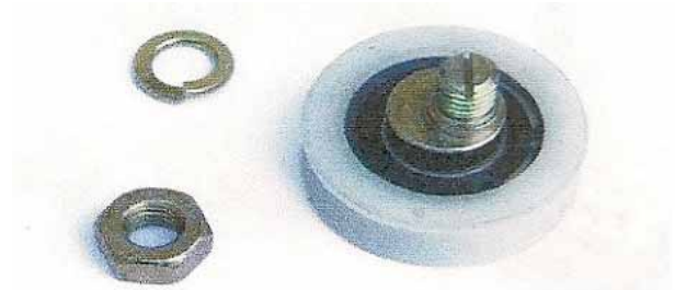
■ ROLDANA Código:53/536 Material: Nylon
